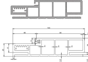
140'lık Kasa 140 mm Frame
