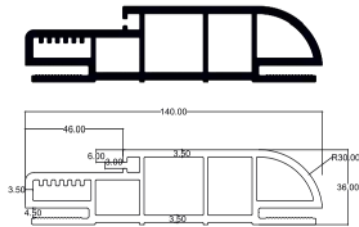
140'lık Kasa 140 mm Frame
