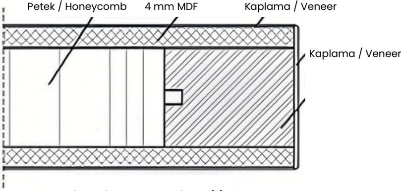
Kaplamalı Kapı Kanadı Kesiti Veneered Door Leaf Section
